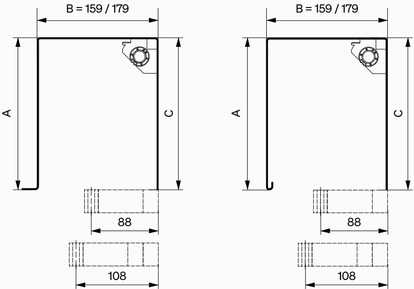
Plech typ F11
