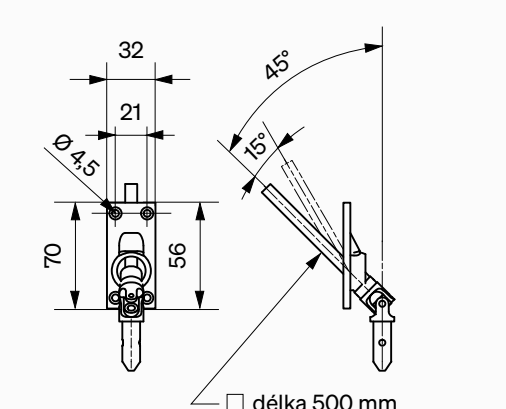
Průchod kliky 45° (8 mm, 4 hran plast) 32×70 mm
