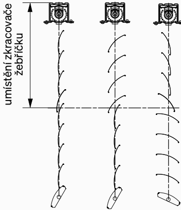
směr dolů mezipoloha směr nahoru
