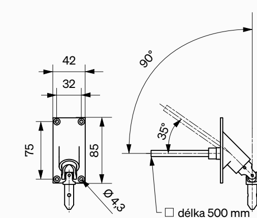
Průchod kliky 90° (8 mm, 4 hran) 42×85 mm
