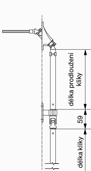
Pomocný kloub kliky
