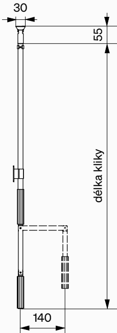
Odnímatelná klika
