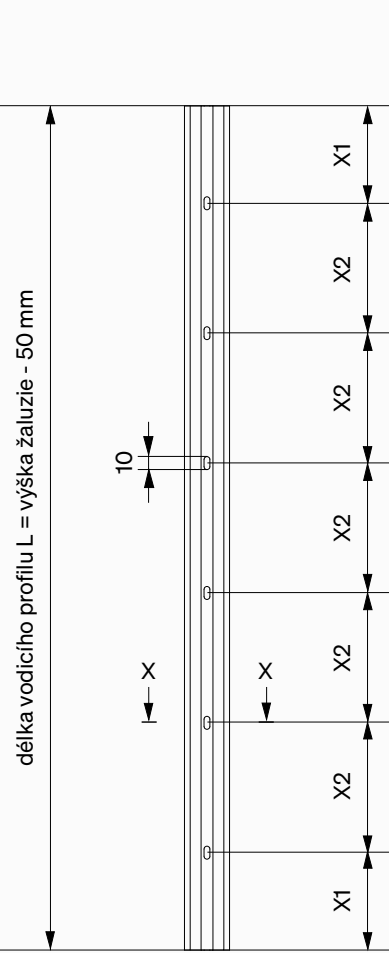
Nedělený vodicí profil
