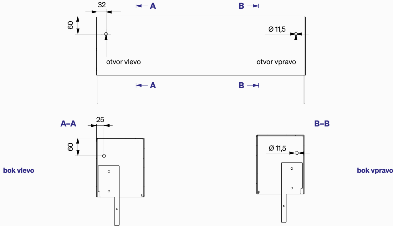
Otvory - zadní strana krycího plechu / pohled z interiéru
