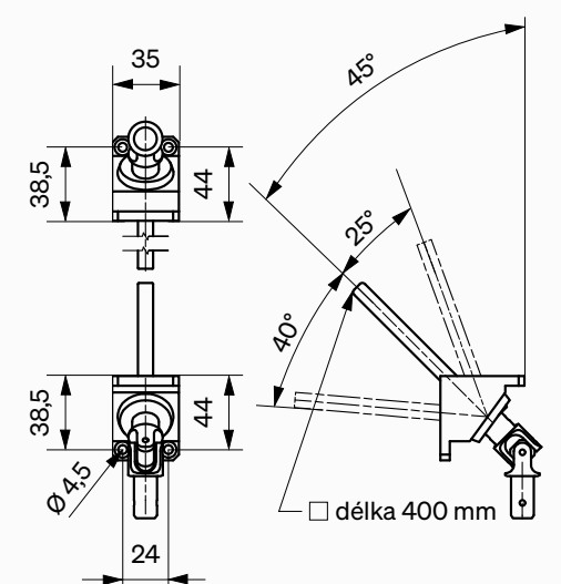
Rohový průchod kliky (8 mm, 4 hran)
