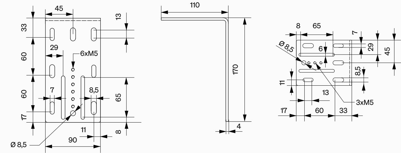
Držák č. 52
