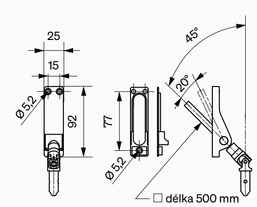
Průchod kliky 45° (8 mm, 4 hran plast) 25×90 mm
