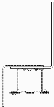
Držák č. 5
