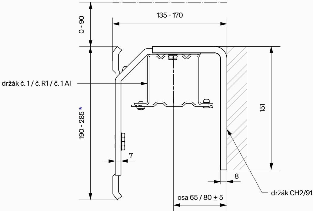
Držák CH3/91
