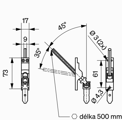
Průchod kliky 45° (6 mm, 6 hran)
