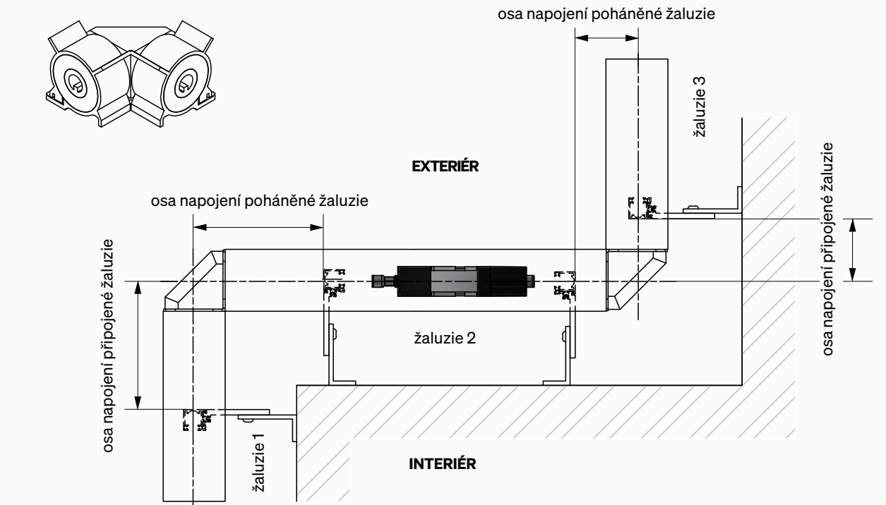
Spojka rohová 90°
