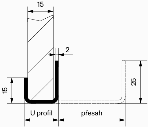
U profil bez izolace
