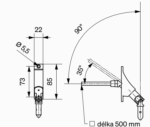
Průchod kliky 90° (8 mm, 4 hran)
