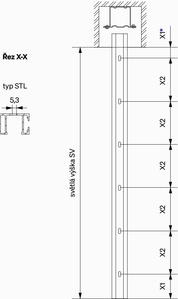
Děrování podle světlé výšky
