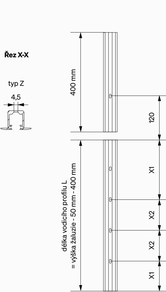
Dělený vodicí profil (dodání ve 2 kusech)
