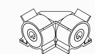
Spojka rohová 90°
