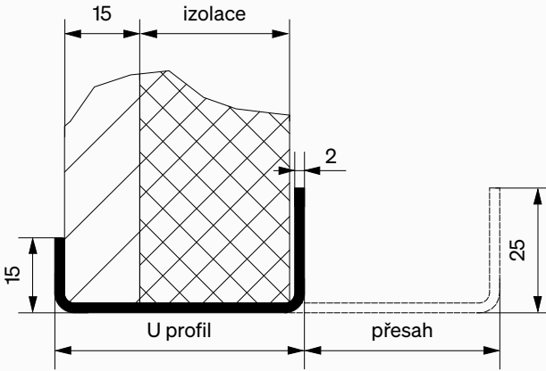
U profil s izolací
