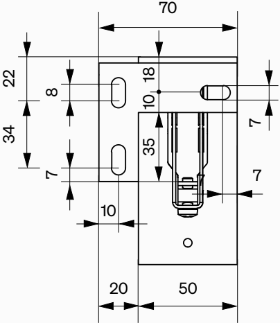
Držák č. 3L
