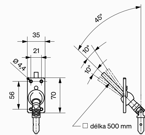
Průchod kliky 45° (8 mm, 4 hran inox) 35×70 mm
