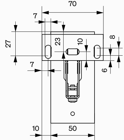
Držák č. 3S *
