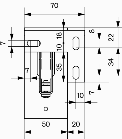
Držák č. 3P
