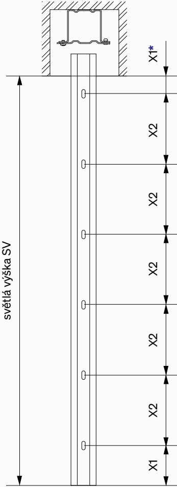
Děrování podle světlé výšky
