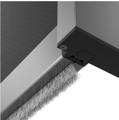
SPODNÍ PROFIL S KARTÁČEM
