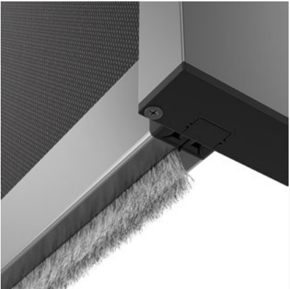
UNTERLEISTE MIT BÜRSTE
